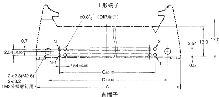
直端子
